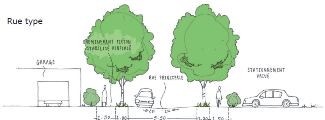
Coupe type voirie principale
